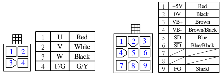
Motor Wiring
